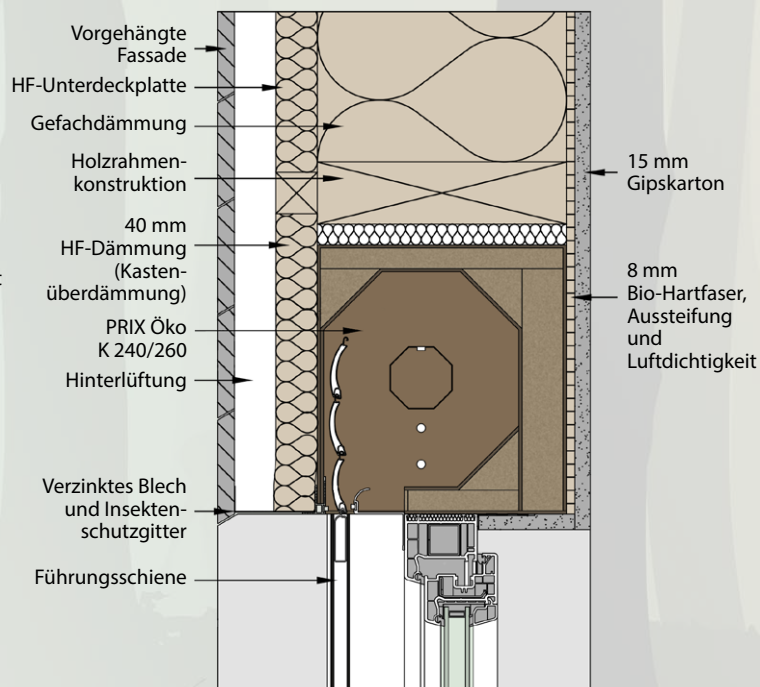
Öko K 240/260 mit VHF
