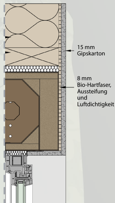
Öko K 260/260 ohne Installationsebene
