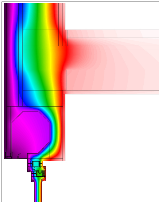
Thermobild PRIX Öko K 260/260
