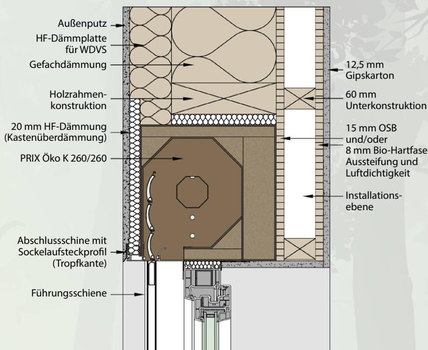
Öko K 260/260 mit Installationsebene
