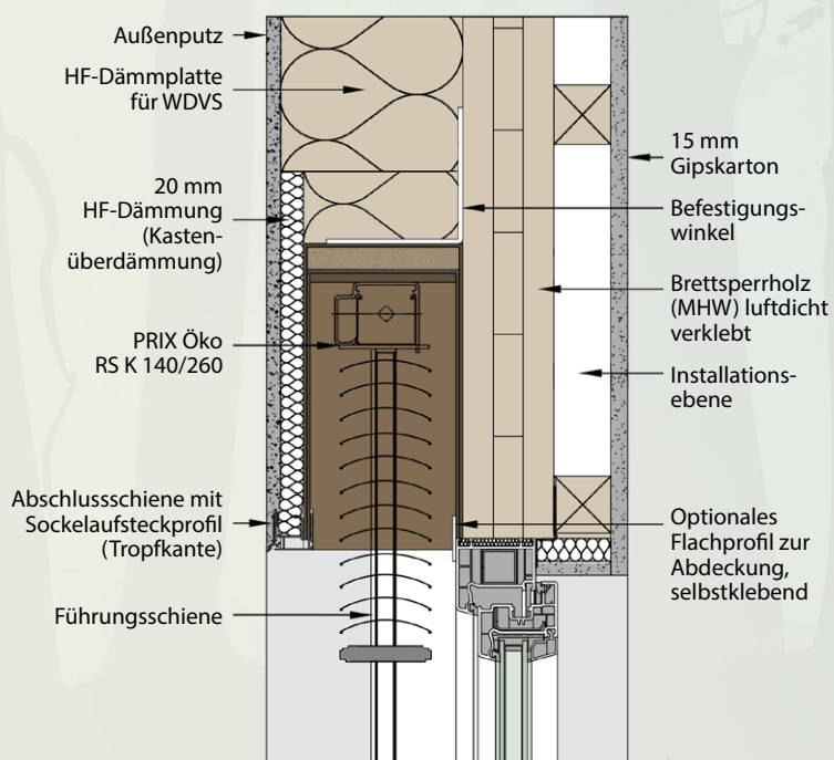
Öko RS K 140/260 als Vorbaukasten
